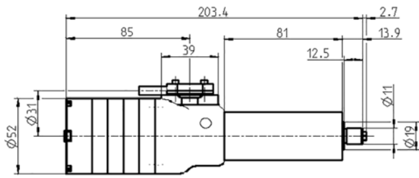
尺寸
