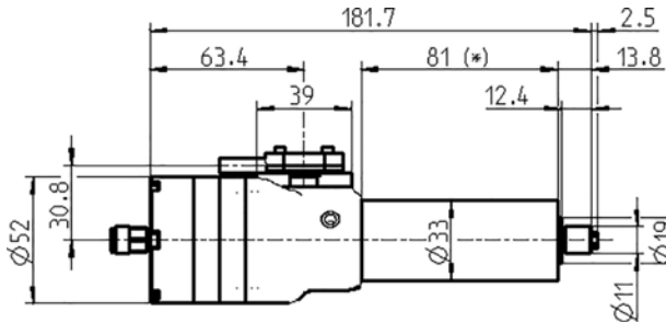
Abmessungen
