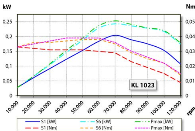
Diagram výkonu Chlazení stlačeným vzduchem
