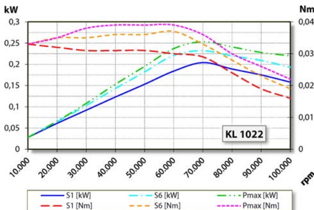
Diagrama de potência Por ar comprimido
