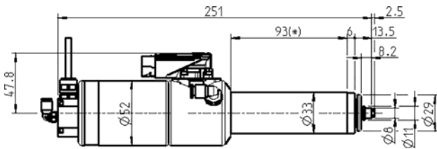
尺寸
