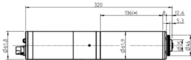
Abmessungen
